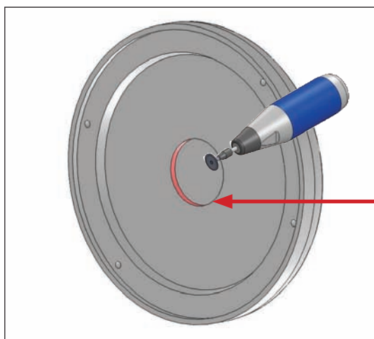
Ord.No.10/23 Trennscheibe Widia disc cutter
