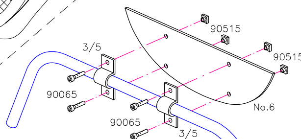
Baugruppe 2 Hinterer Kufenbügelspann
