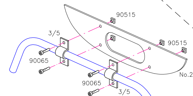
Baugruppe 1 Hauptträgerplatte mit vorderem Kufenbügel
