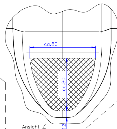
Baugruppe 2 Hinterer Kufenbügelspann
