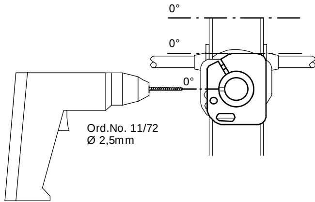
Ansicht Z
