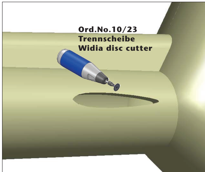
Ord.No.10/23 Trennscheibe Widia disc cutter
